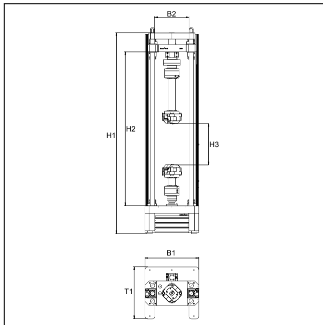
Zeichnung: Z600E – Prüfung an Faserverbundwerkstoffen
